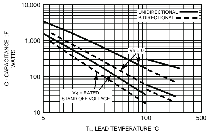
FIG. 6 - CAPACITANCE
